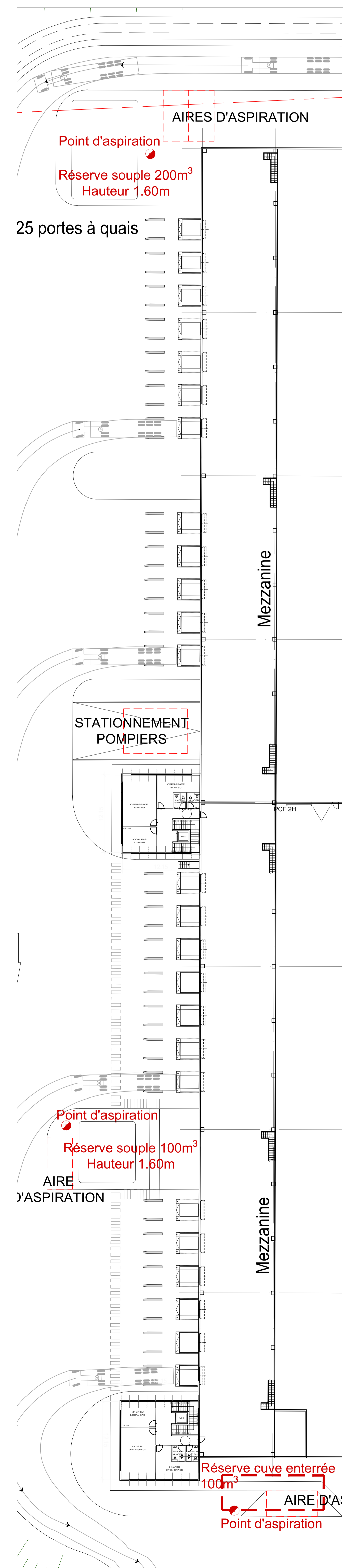
PLAN MEZZANINE OUEST
